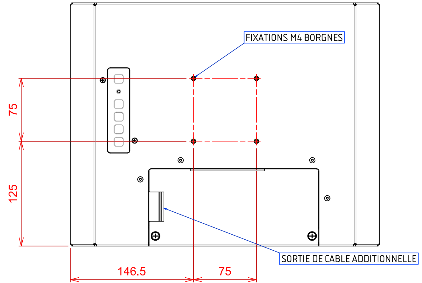
VUE ARRIERE
